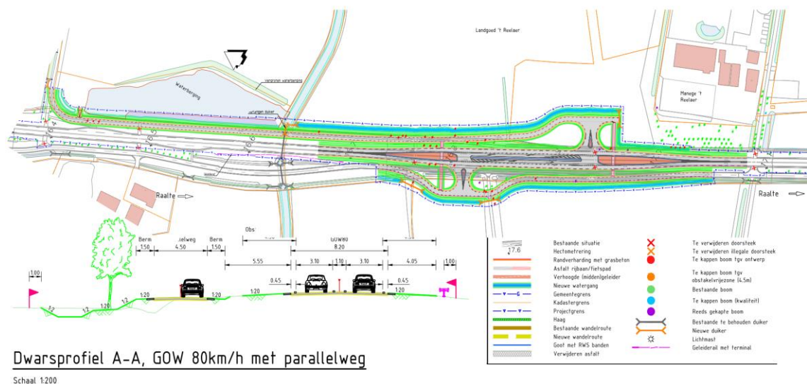
Figuur: Ontwerp aanleg bajonetkruising en nieuwe oostelijke parallelweg
